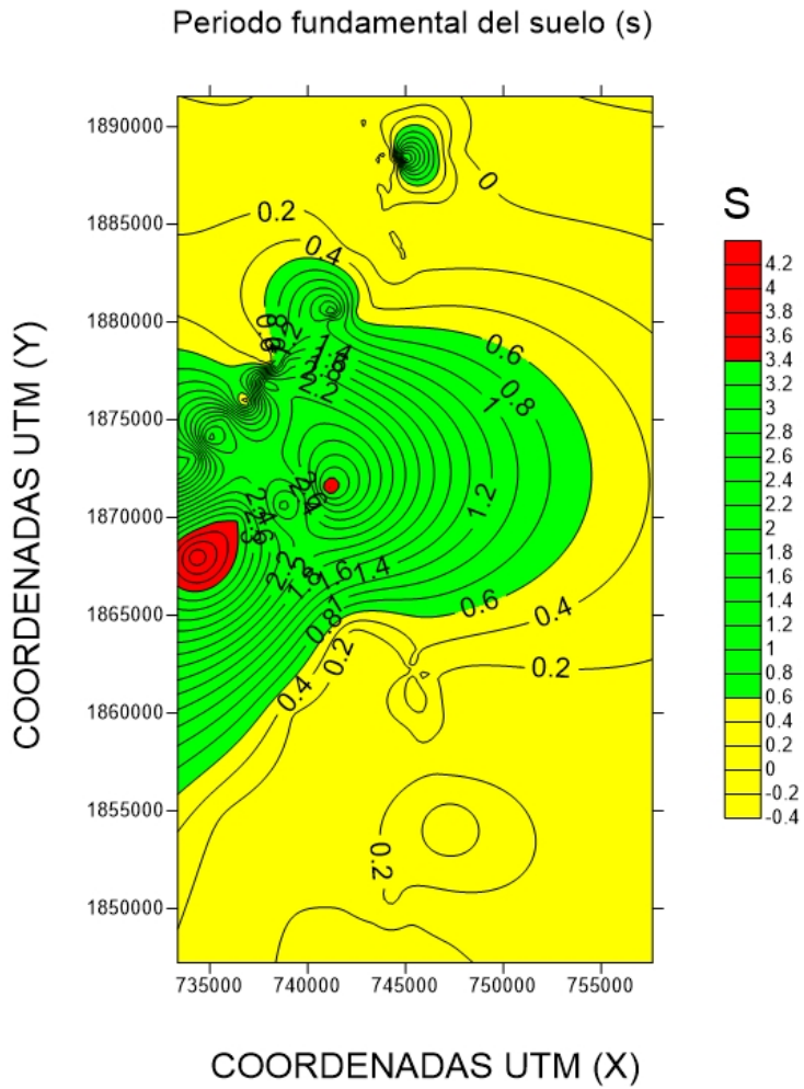
Figura 4.13. Periodo fundamental del suelo (s)
