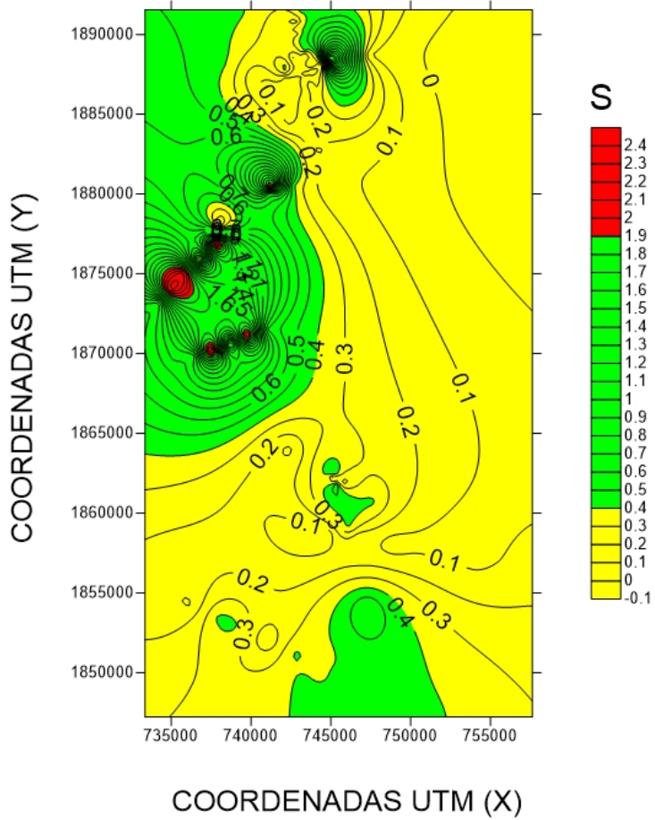
Figura 4.15. Periodo estructural con mayor aceleración absoluta (s)
