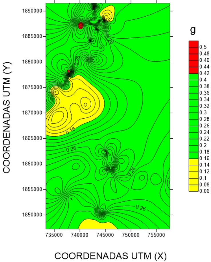
Figura 4.16. Máxima aceleración del terreno
