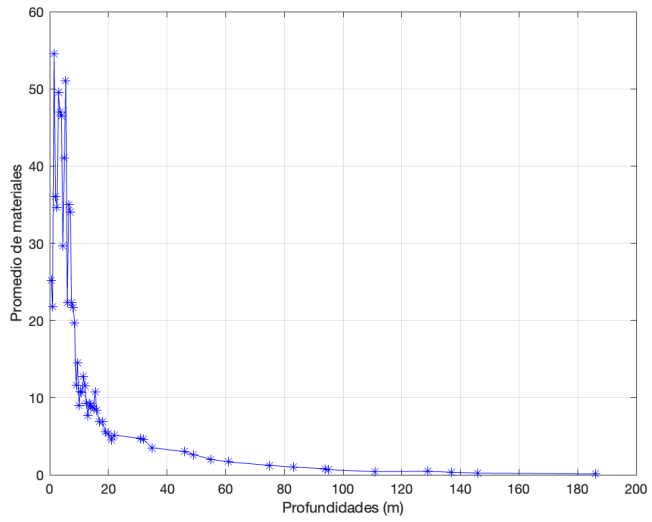
Figura 4.7. Promedio de los materiales por profundidad
