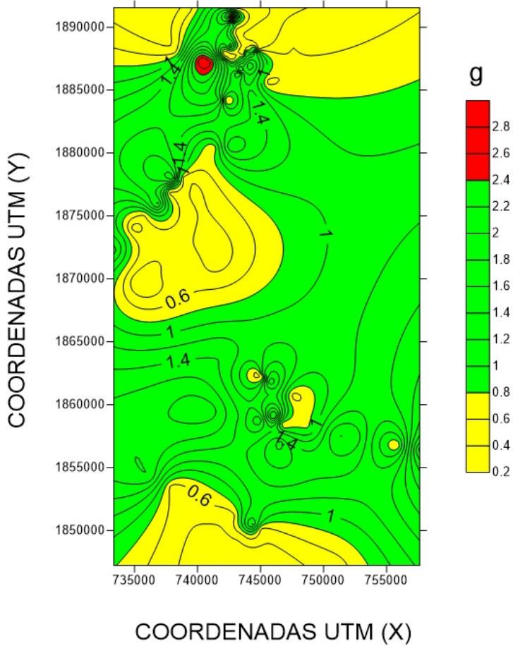
Figura 4.14. Aceleración absoluta del periodo estructural anterior
